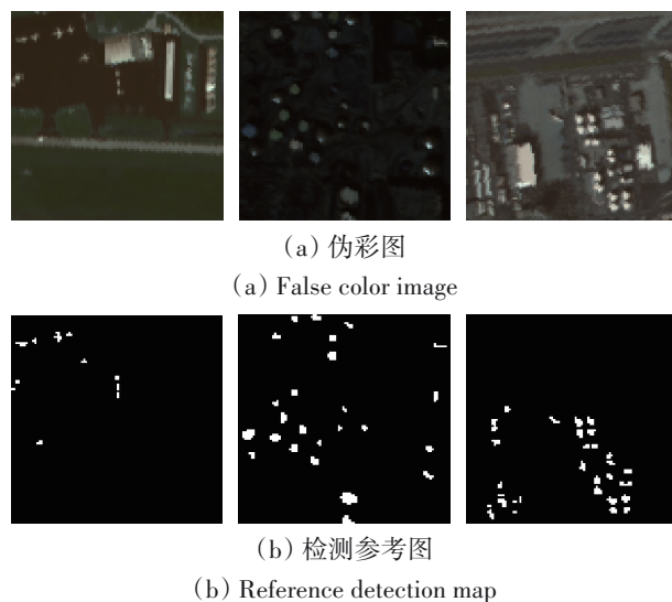
图3 ABU数据集
