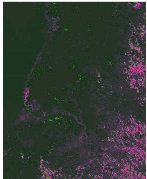
图5 2007-08-22 云及其阴影地域增强图像
